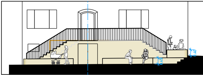
ANSICHT M 1:200
