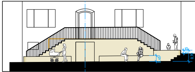
ANSICHT M 1:200
