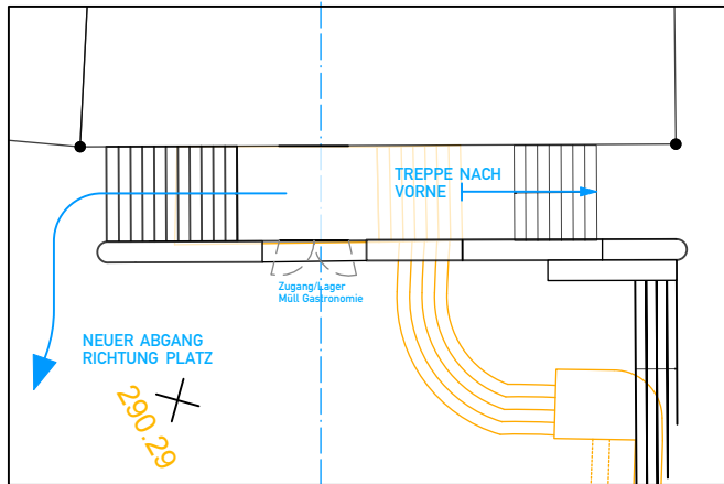
GRUNDRISS M 1:200
